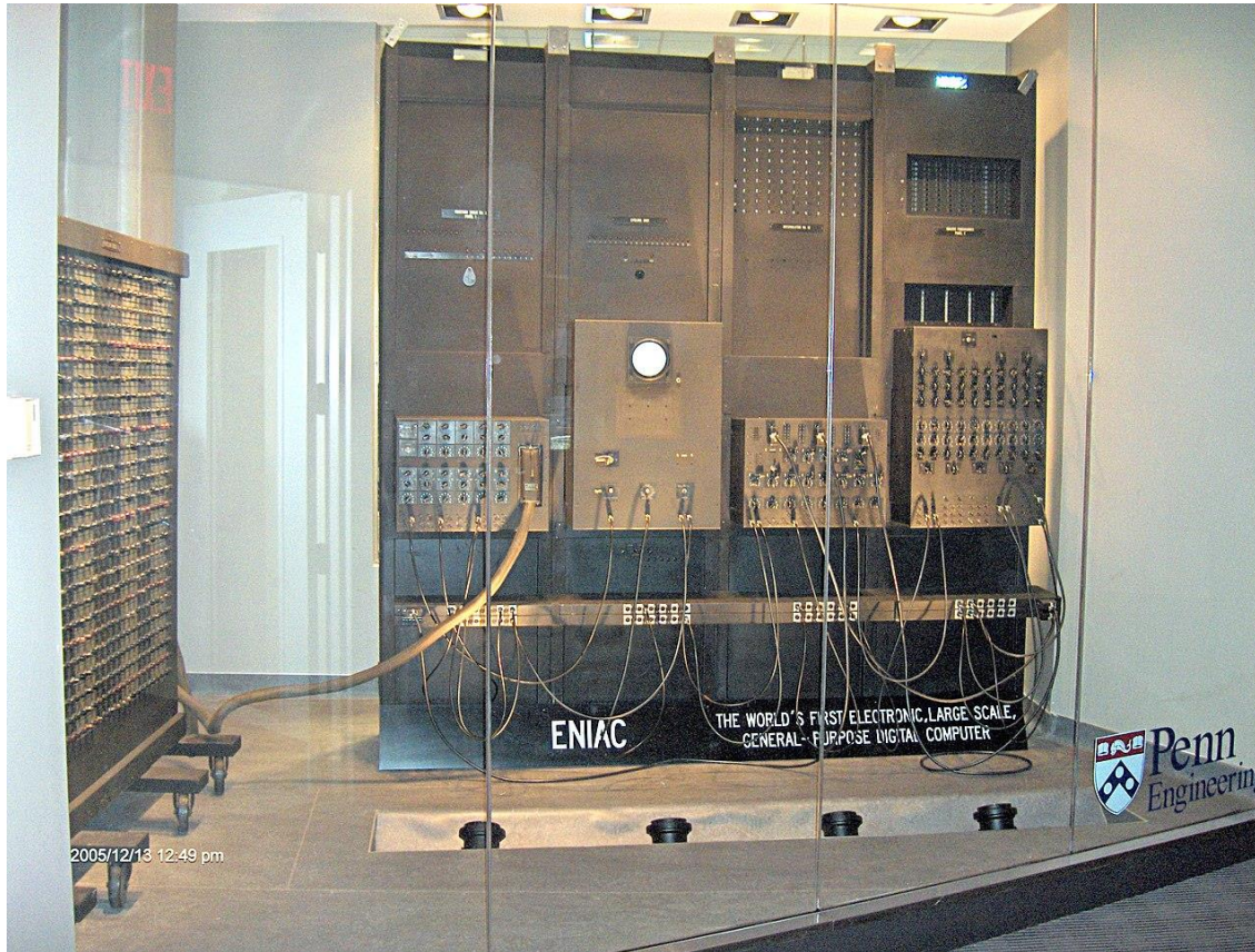
ENIAC, 1943
